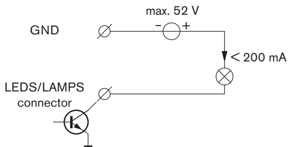
Ábra 5.27: Lámpák csatlakoztatása
