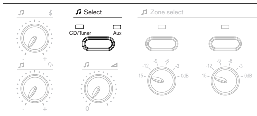
Ábra 7.3: Háttérzene forrásának kiválasztása
