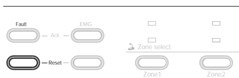
Ábra 7.20: Fault reset (Hiba törlése) gomb
