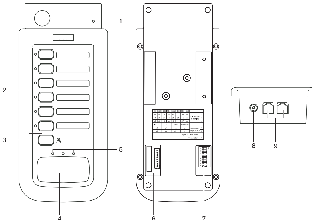
Ábra 3.7: Bemondópult felső és alsó nézete
