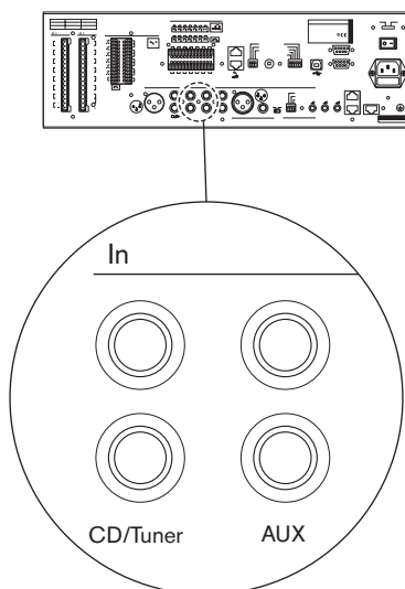
Ábra 5.14: Háttérzene-bemenetek
