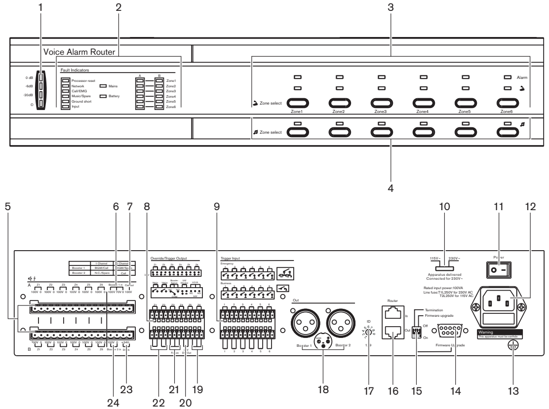
Ábra 3.4: A vészhangosítási rendszer zónabővítőjének elülső és hátsó nézete
