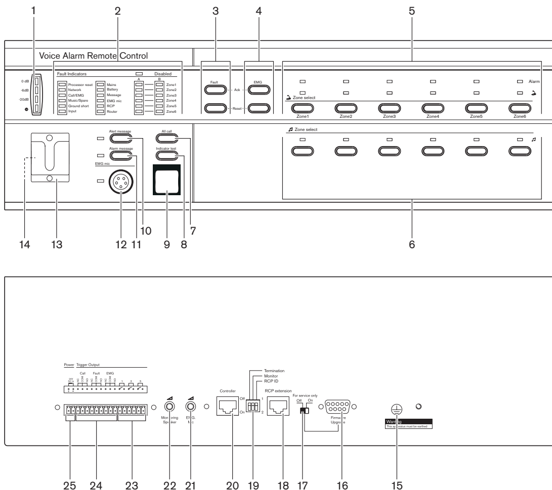
Ábra 3.9: A vészhangosítási rendszer távvezérlőjének elülső és hátsó nézete
