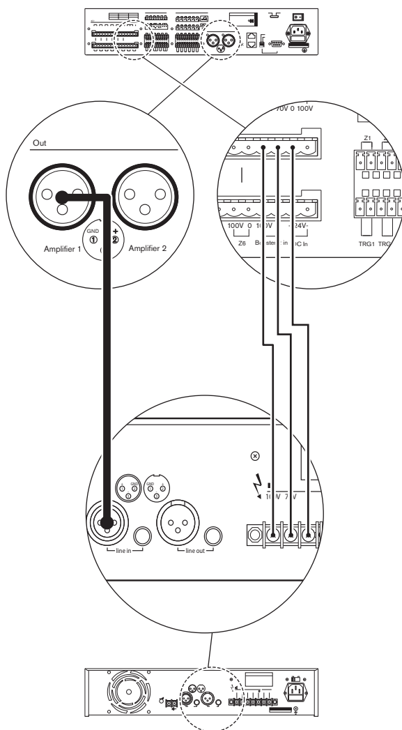
Ábra 5.21: 1. külső teljesítményerősítő csatlakoztatása
