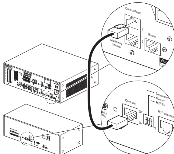
Ábra 5.5: Távvezérlő csatlakoztatása
