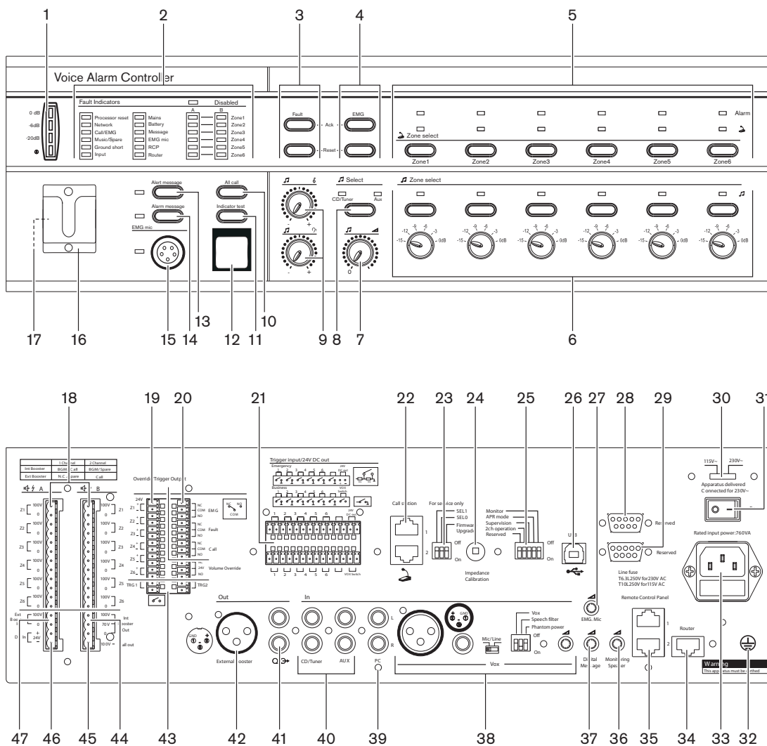
Ábra 3.2: A vészhangosítási rendszer vezérlőjének elülső és hátsó nézete
