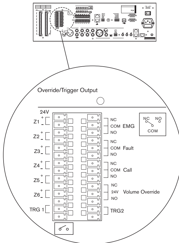
Ábra 5.7: Felülvezérlés kimenetek
