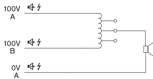
Ábra 5.10: 3-vezetékes hangerő-felülvezérlés
