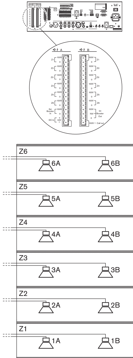
Ábra 5.6: Hangszórózónák csatlakoztatása
