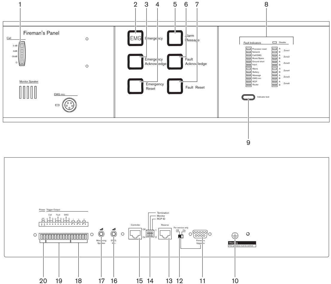
Ábra 3.13: Tűzjelző központ elülső és hátsó nézete
