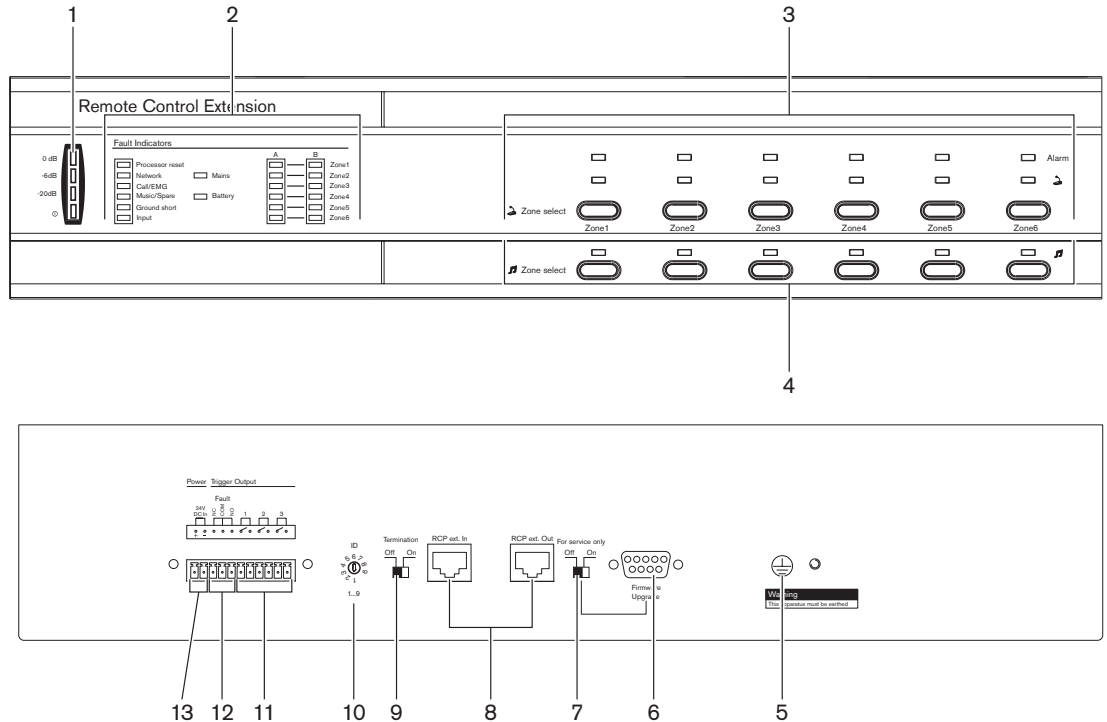
Ábra 3.11: A távvezérlő bővítőjének elől- és hátulnézete
