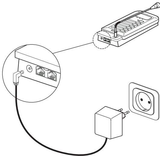
Ábra 5.23: Tápellátás csatlakoztatása
