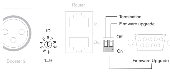
Ábra 6.6: A zónabővítő beállításai
