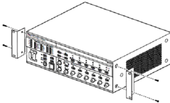
Ábra 4.1: Tartókonzolok a rack szekrénybe történő szereléshez
