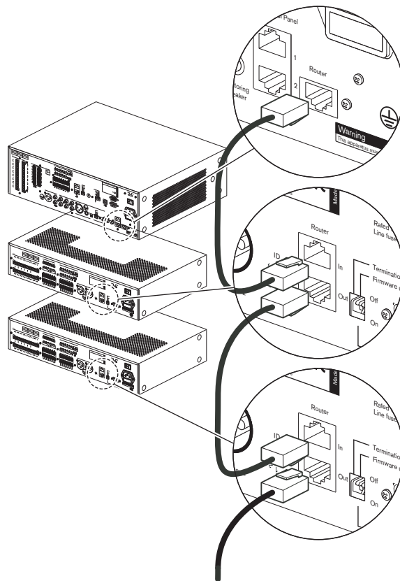
Ábra 5.3: Zónabővítők csatlakoztatása
