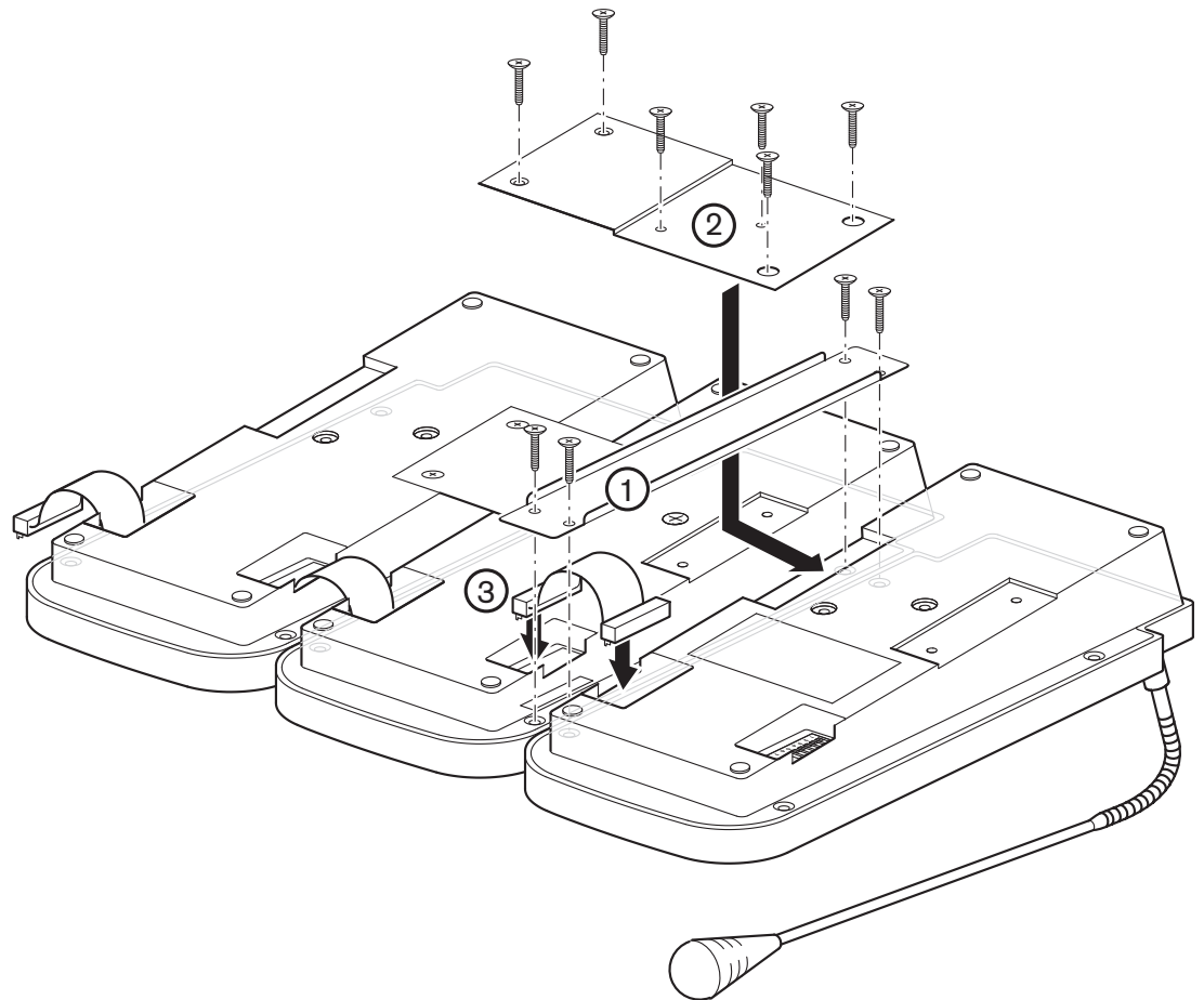
Ábra 4.2: A bemondópult billentyűzeteinek csatlakoztatása
