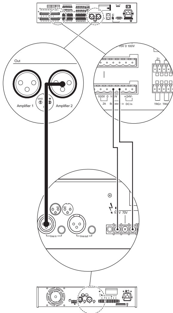
Ábra 5.22: 2. külső teljesítményerősítő csatlakoztatása
