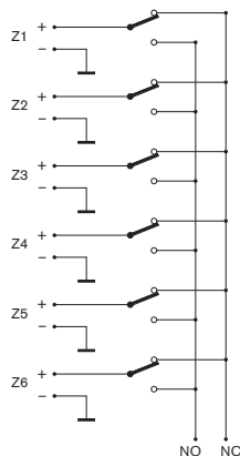
Ábra 5.8: Hangerő-felülvezérlési csatlakozók
