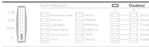
Ábra 6.2: Disabled (Letiltva) visszajelző
