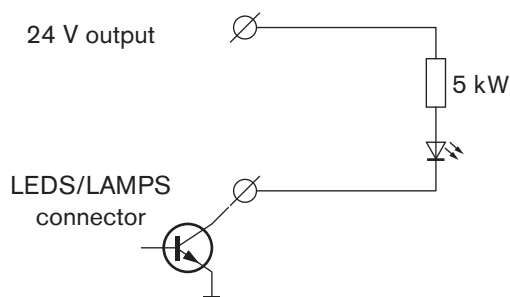
Ábra 5.26: LED-ek csatlakoztatása
