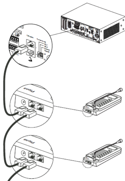
Ábra 5.2: A bemondópultok csatlakoztatása
