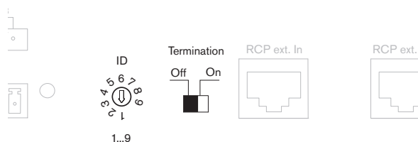
Ábra 6.9: A távvezérlő beállításai
