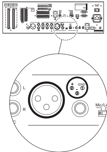
Ábra 5.12: Mikrofon-/vonalbemenet VOX funkcióval
